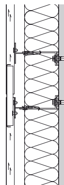
Przekrój
