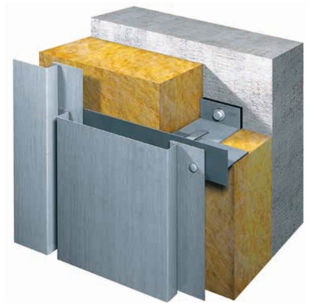
Podkonstrukcja dwuelementowa
