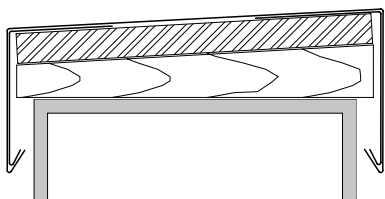
RHEINZINK-Obróbki attyk
