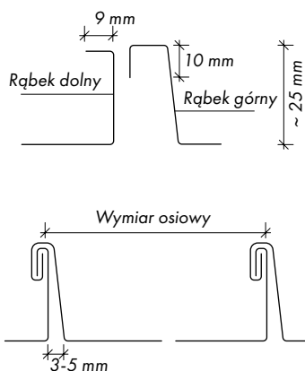
RHEINZINK-podwójny rąbek stojący
