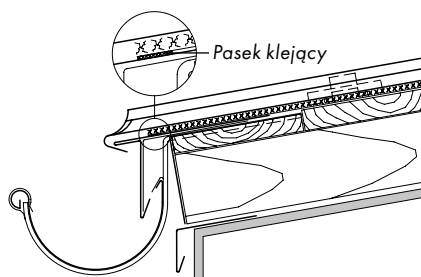
Pas okapowy z matą strukturalną
