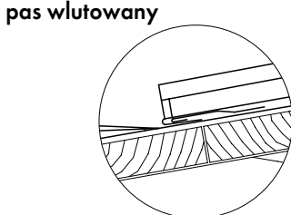
Optymalne wykonanie: dodatkowy pas włutowany
