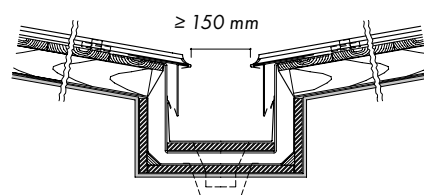
Rynna wewnętrzna skrzynkowa z wyklejaną rynną zabezpieczającą
