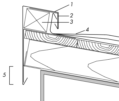
Kalenica dachu jednospadowego na listwę
