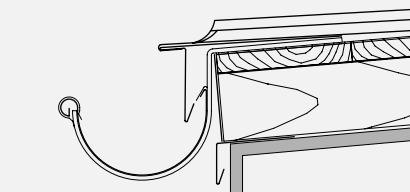
Okap na deskowaniu – niewłaściwe wykonanie detalu
