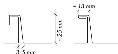
RHEINZINK-System rąbka kątownego
