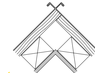
Narożnik budynku
